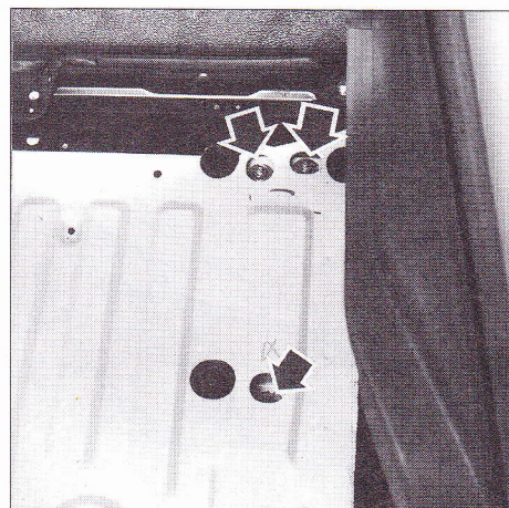
Vis de fixation du train arrière à la caisse.
