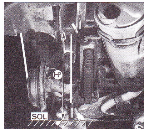
Mesure de la cote H3.
