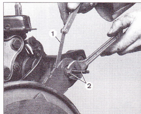
Repose du levier droit de barre stabilisatrice. 1. Cale d'épaisseur 1 mm - 2. Outil Peugeot 0908S1, S2 et S3.
