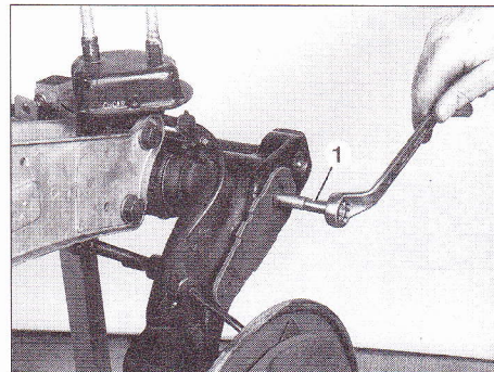
Dépose d'un levier de barre stabilisatrice avec la vis (1) Peugeot 0908R.
