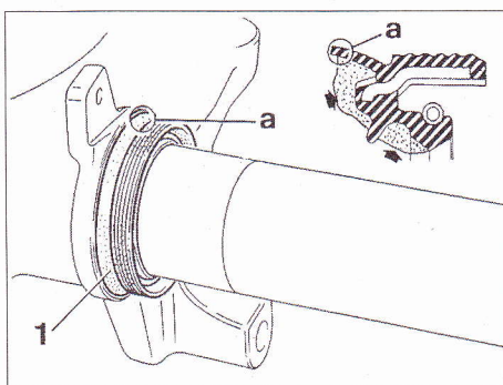
Repose d'un bras de suspension : mise en place de la bague d'étanchéité. 1. Bague - a. Lèvre extérieure.
