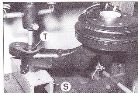
Extraction de l'axe du bras de suspension et de la coupelle. T. Tampon - S. Appui.
