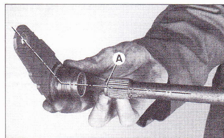
Assemblage du levier et de la barre stabilisatrice. Aligner le repère (A) avec la boutonnière.
