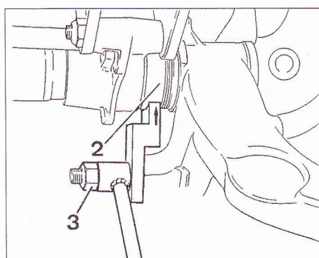
Repose d'un bras de suspension. 2. Manchon - 3. Écrou.
