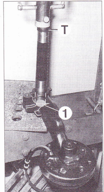
Mise en place de l'axe du bras de suspension et de la coupelle. 1. Cale Peugeot 0526U - T. Tampon.
