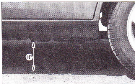
Mesure de la cote H2.
