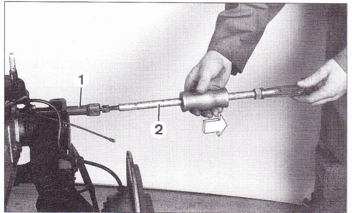
Dépose d'une barre de torsion à l'aide d'un extracteur à inertie. 1. Barre de torsion - 2. Extracteur.
