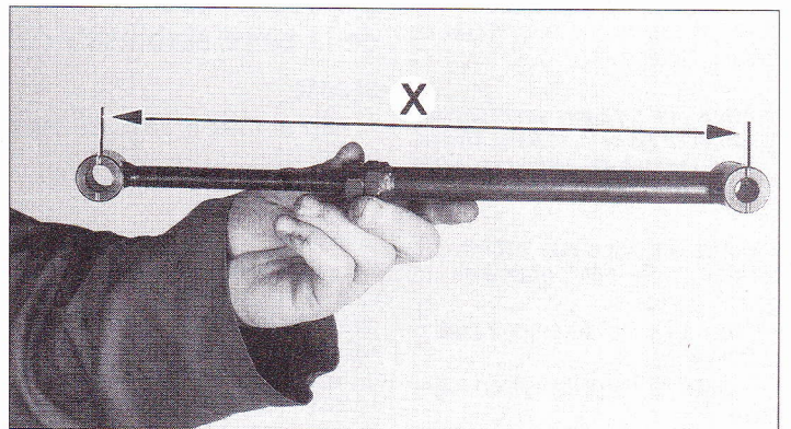
Mesure de la longueur " X " du faux amortisseur.
